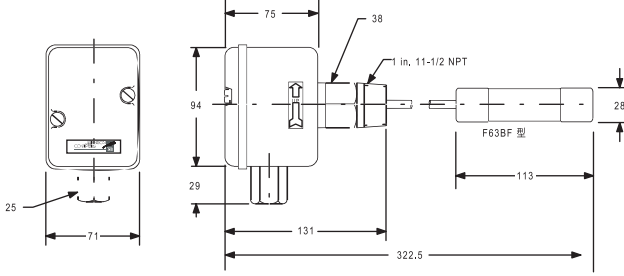
尺寸 (mm)
